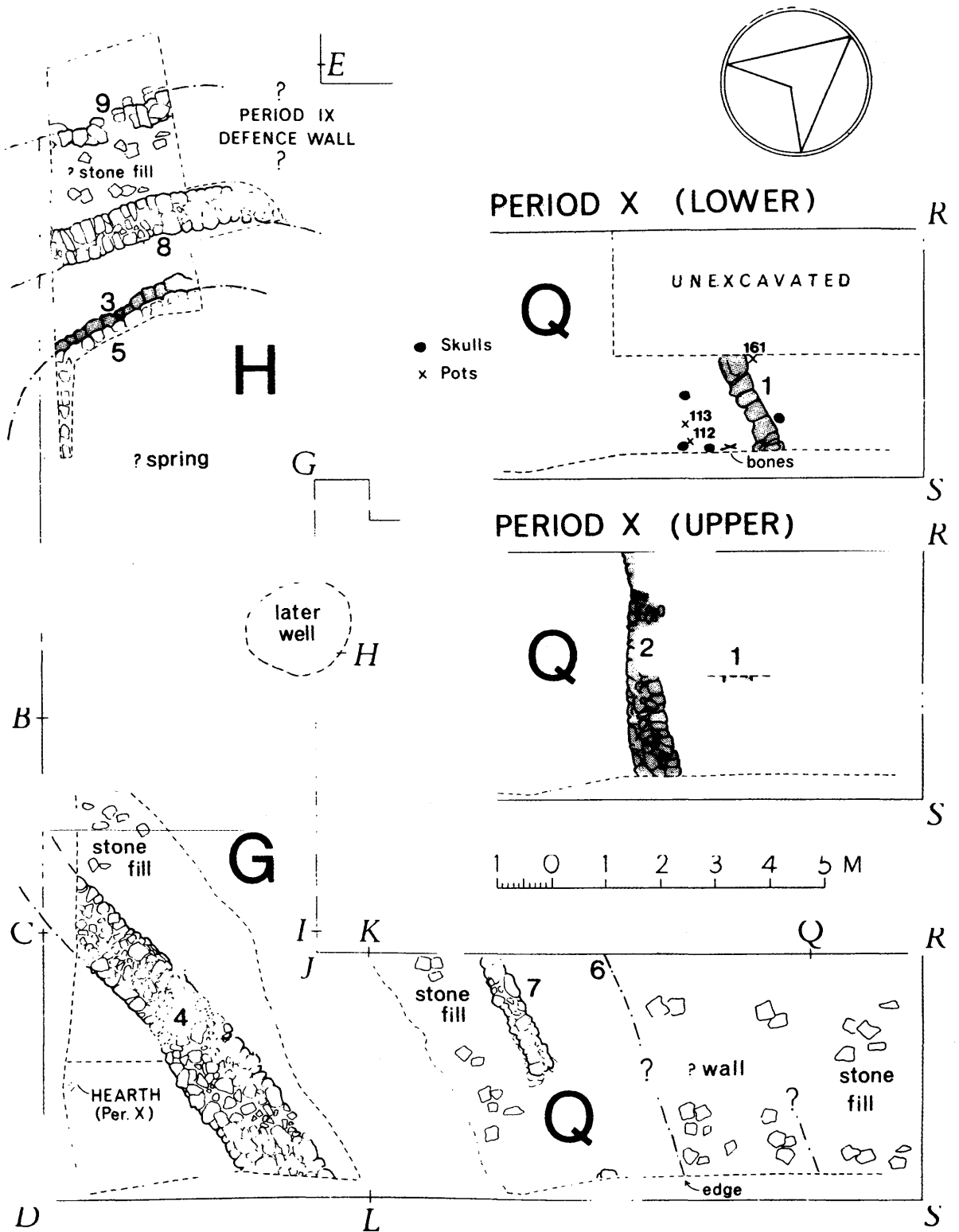
Ειχ. 1. Εμποριό Χίου. Λιθόκτιστοι περιβόλοι των φάσεων X και IX (κατά Hood 1982, ειχ. 52).
