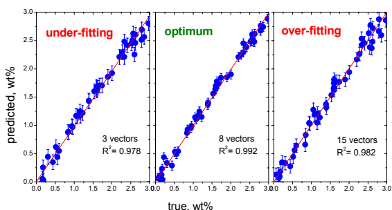
Σχήμα 5. Συσχετισμός προβλεπόμενων και πραγματικών τιμών της συγκέντρωσης του συστατικού \delta με 3, 8 και 15 ανύσματα βάσης. Είναι φανερή η βελτιστοποίηση του συσχέτισμού με ενδιάμεσο αριθμό ανυσμάτων βάσης (πρβλ. Σχ. 4).
