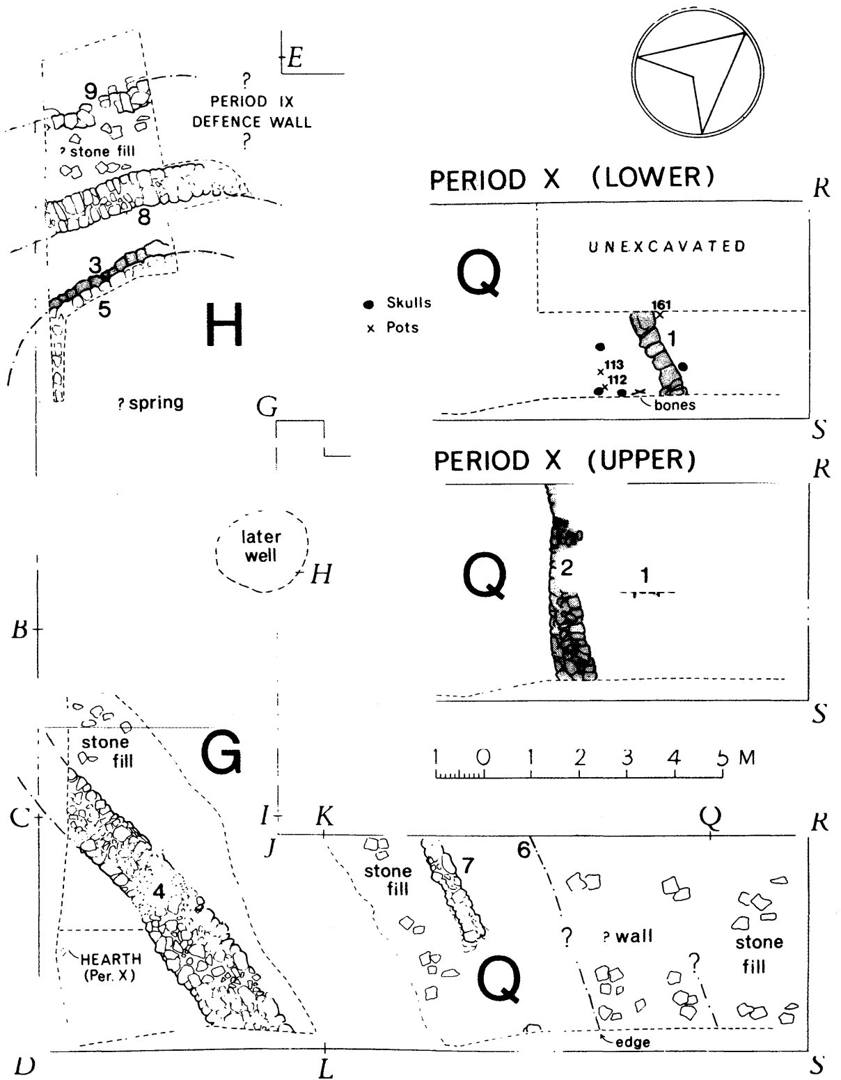
Εικ. 1. Εμποριό Χίου. Λιθόκτιστοι περιβόλοι των φάσεων X και IX (κατά Hood 1982, εικ. 52).
