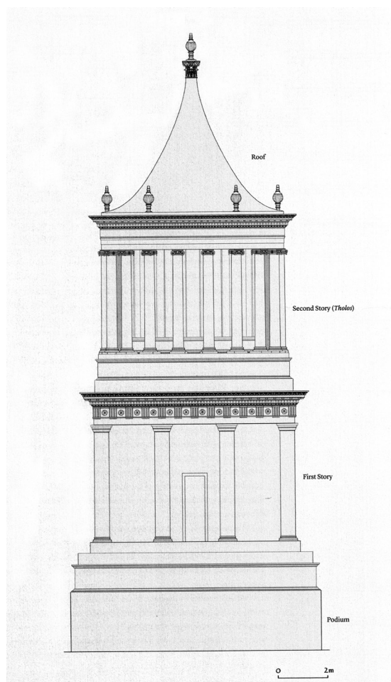
Fig. 17. Hérodon, restitution du tombeau d'Hérode par E. Netzer (d'après ROZENBERG, MNEVORAH 2013, 257).
