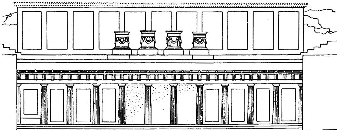
Fig. 13. Lindos (Grèce), restitution de la façade rupestre de l'Archokratéion (d'après KÄHLER 1971, fig. 10).
